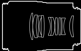
レンズ構成図 < 9群 10枚 >
