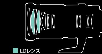
レンズ構成図 < 11群14枚 >
